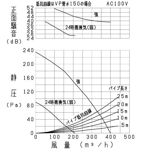
VD-20ZLC 13 -IN/P-Q・騒音特性
