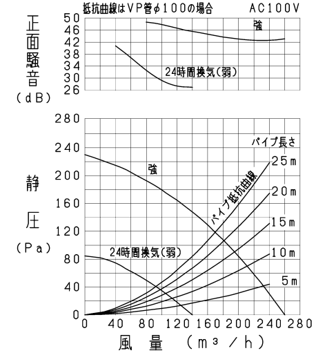
VD-18ZLSC 13 -IN/P-Q・騒音特性
