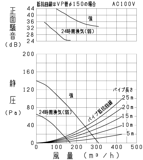
VD-18ZLC 13 -IN/P-Q・騒音特性
