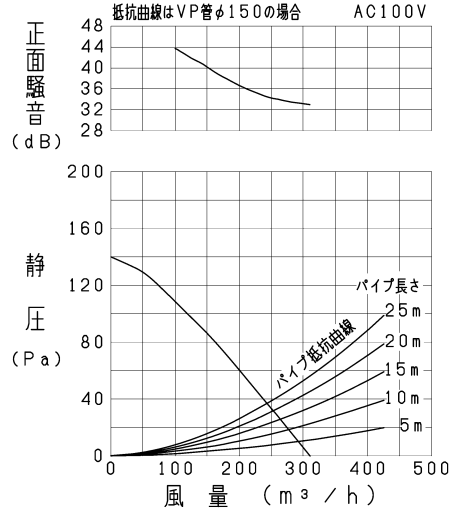
VD-18ZC 13 -IN/P-Q・騒音特性
