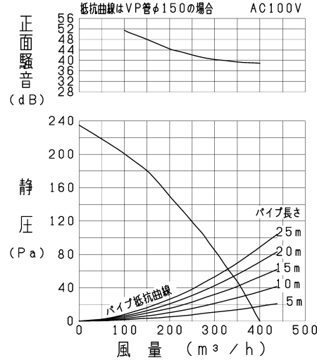
VD-20ZC 13 -IN/P-Q・騒音特性
